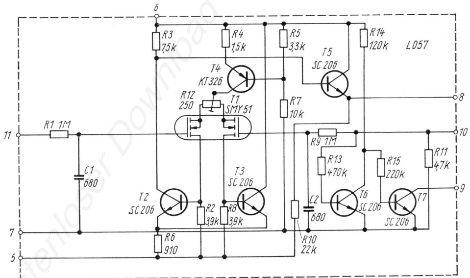
Universal-Kurzzeitmeßgerät Typ MT 10 Leiterplatte L 057
