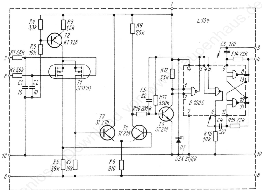
Universal-Kurzzeitmeßgerät Typ MT 10 - Leiterplatte L 104
