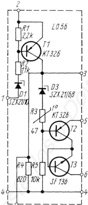
Universal-Kurzzeitmeßgerät Typ MT 10 Leiterplatte L 056
