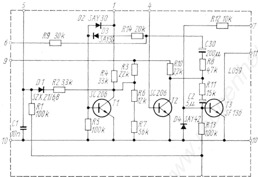
Universal-Kurzzeitmeßgerät Typ MT 10, Leiterplatte L 059
