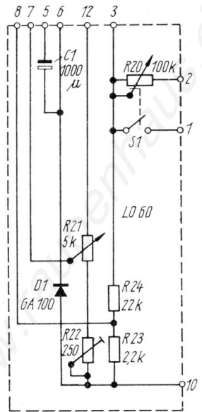
Universal-Kurzzeitmeßgerät Typ MT 10 Leiterplatte L 060/2
